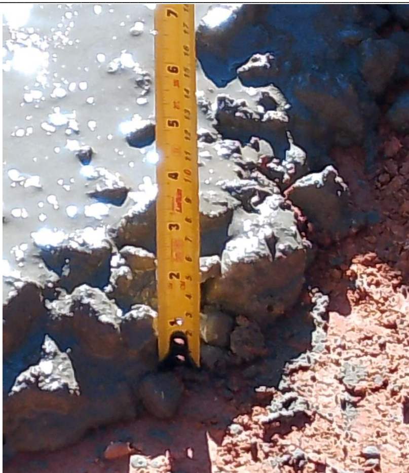
ESPESSURA DA BASE DE DRENAGEM DE 4CM
