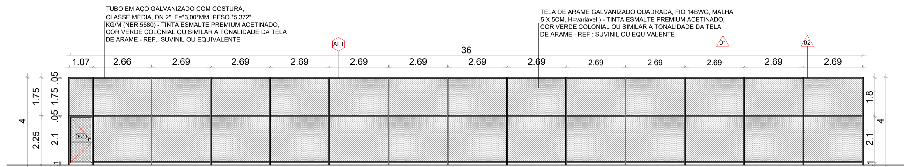
ALAMBRADO AL1 - ELEVÇÃO 04 ESCALA 1/100
