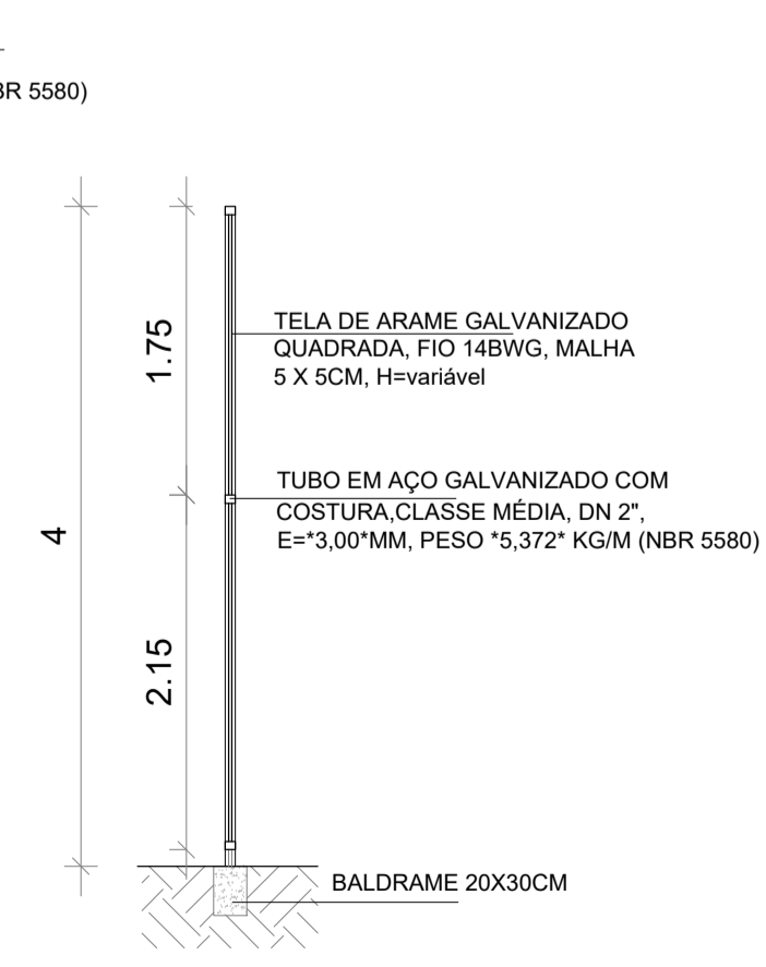
DETALHE TÍPICO - CORTE ALAMBRADO GALVANIZADO ESCALA 1/50
