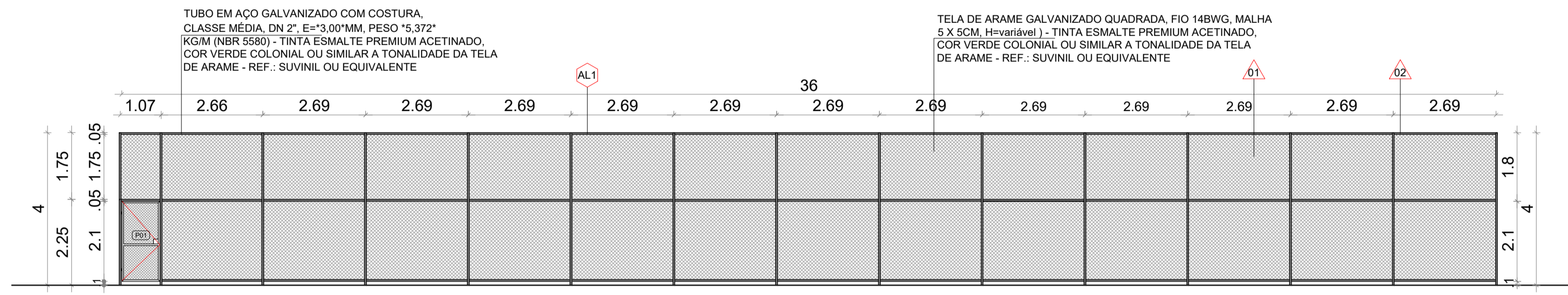
ALAMBRADO AL1 - ELEVÇÃO 02 ESCALA 1/100
