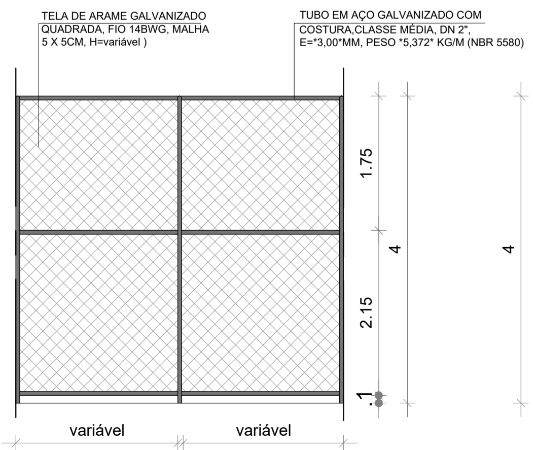
DETALHE TÍPICO - FRONTAL ALAMBRADO GALVANIZADO ESCALA 1/50
