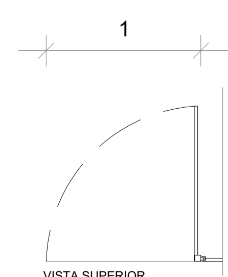
P01 - PORTÃO ACESSO CAMPO ESCALA 1/25
