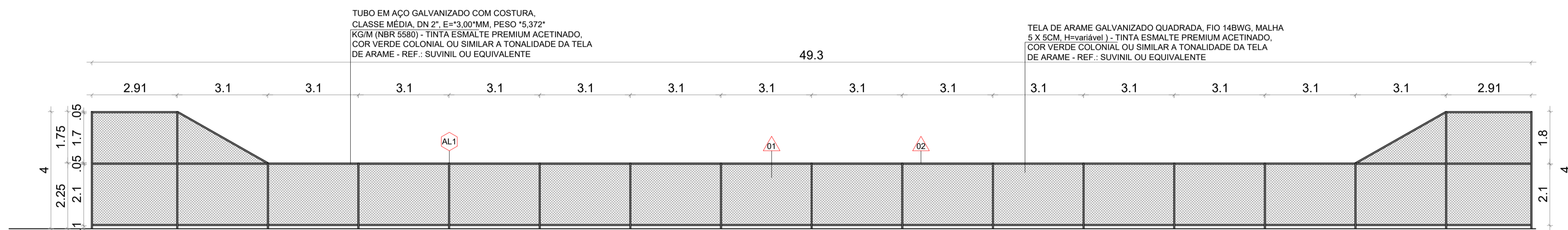
ALAMBRADO AL1 - ELEVÇÃO 03 ESCALA 1/100
