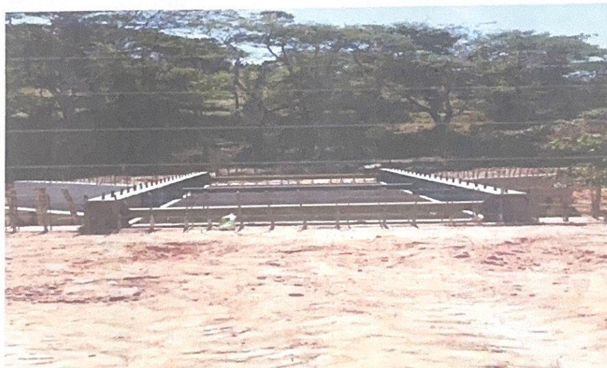
FIGURA 2 – LONGARINAS E TRANSVERSINAS PRONTAS
